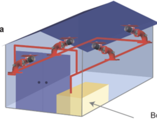
Спринклерная установка пожаротушения со смачивателем «Аквафом СМ»
