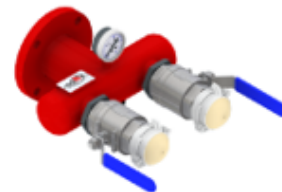
Узел подключения пожарной техники, УПТ
