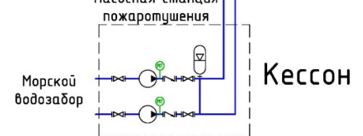
Насосная станция пожаротушения
