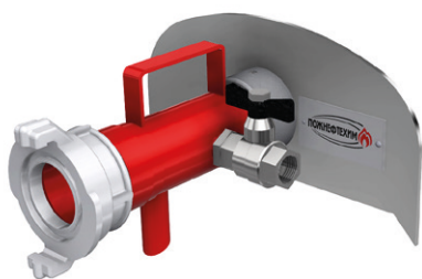
Насадок пожарный НП-III/50П для водяных завес
