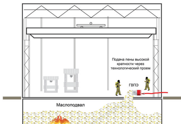
СХЕМА 2. Подача пены высокой кратности через технологический проем в маслоподвал
