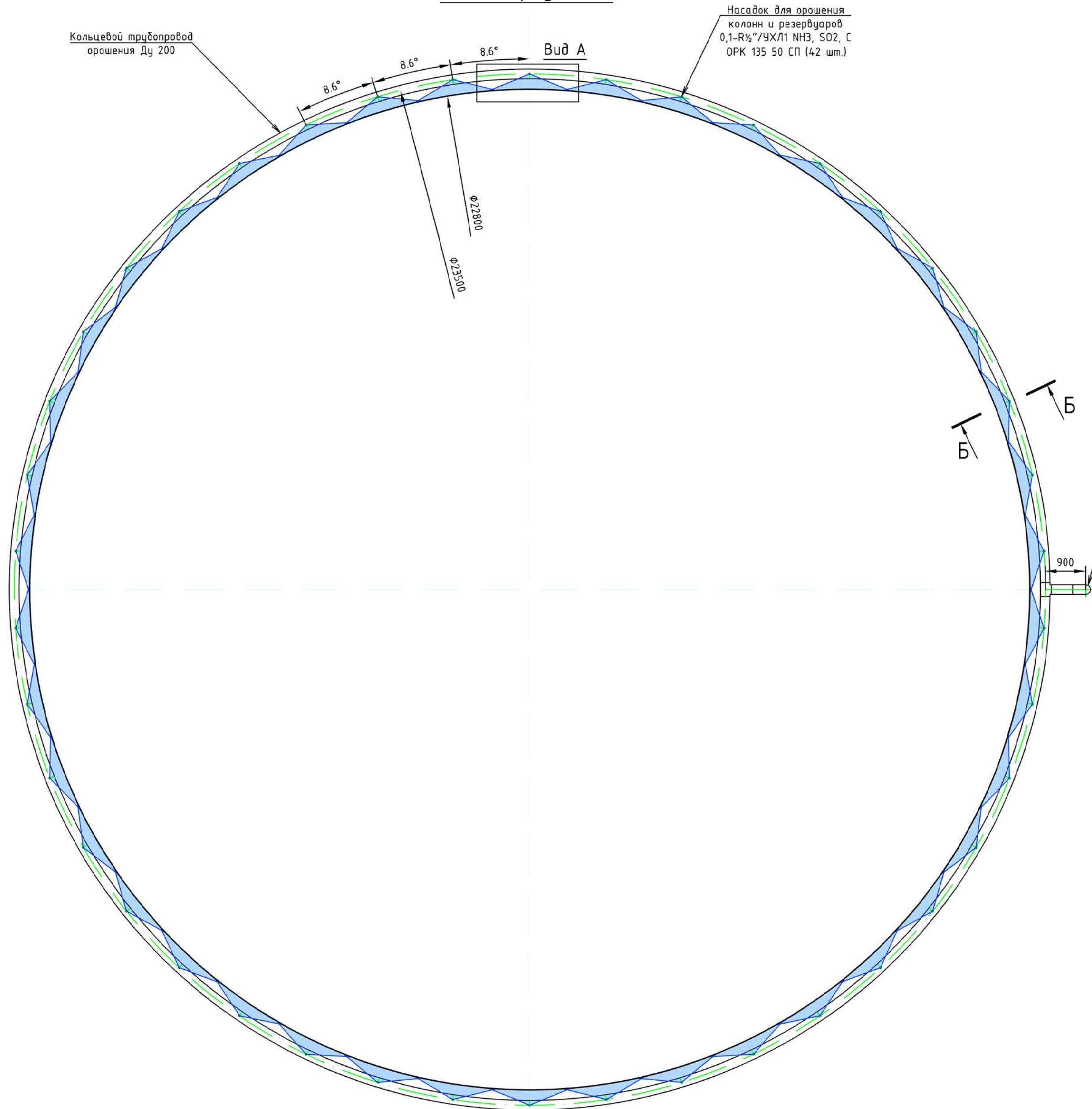
Вид сверху (1:75)
