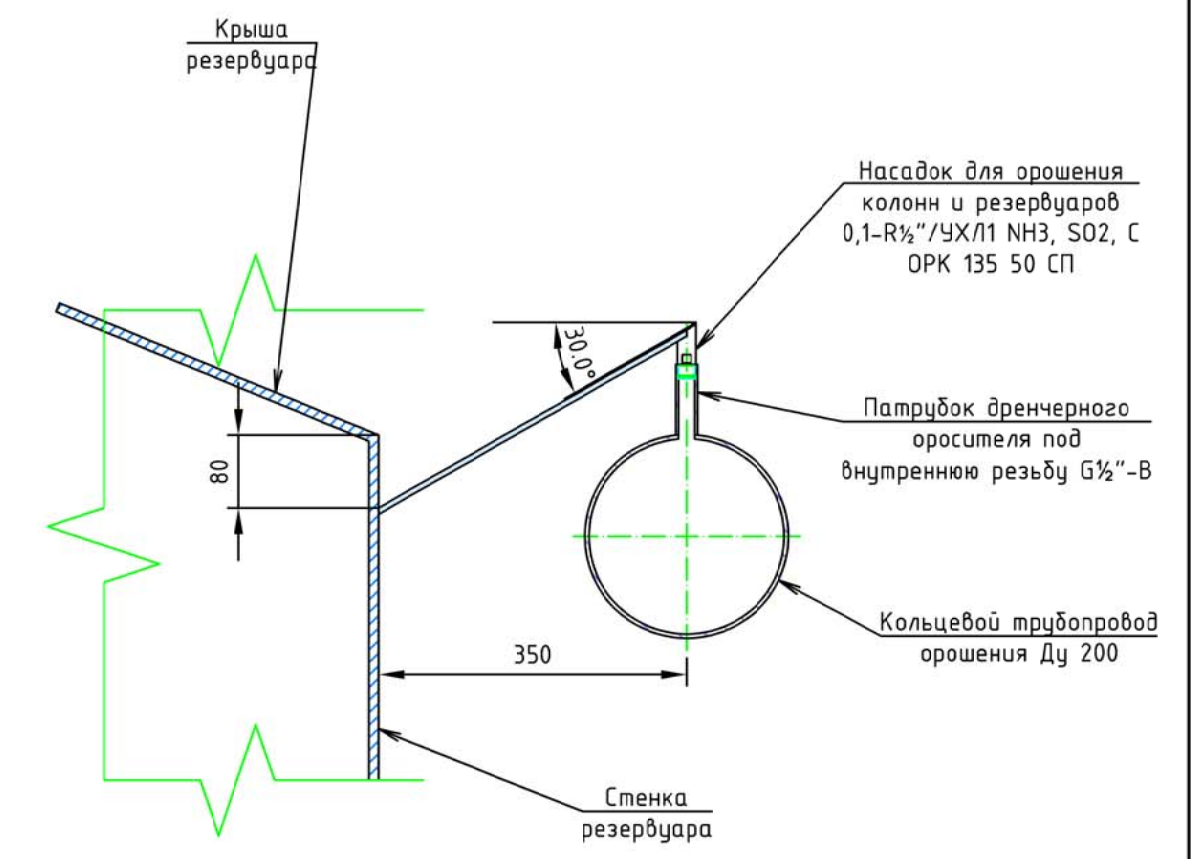
Разрез Б-Б (1:8)
